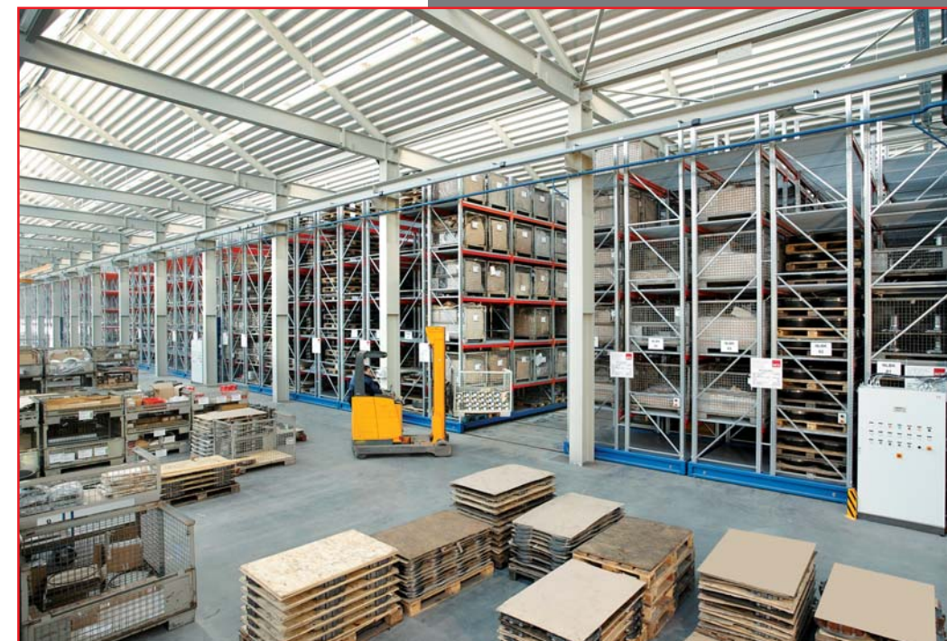
Die neue Verschieberegalanlage im Werk Kocherwiesen ist mit 4.300 Palettenplätzen auf einer Fläche von 1.170 qm die größte von den insgesamt rund 20 META MULTIBLOC Anlagen bei Kessler + Co.
